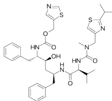
Figure 4: Ritonavir.
