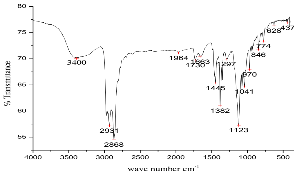
Appendix 2: IR Spectrum of CP-1.
